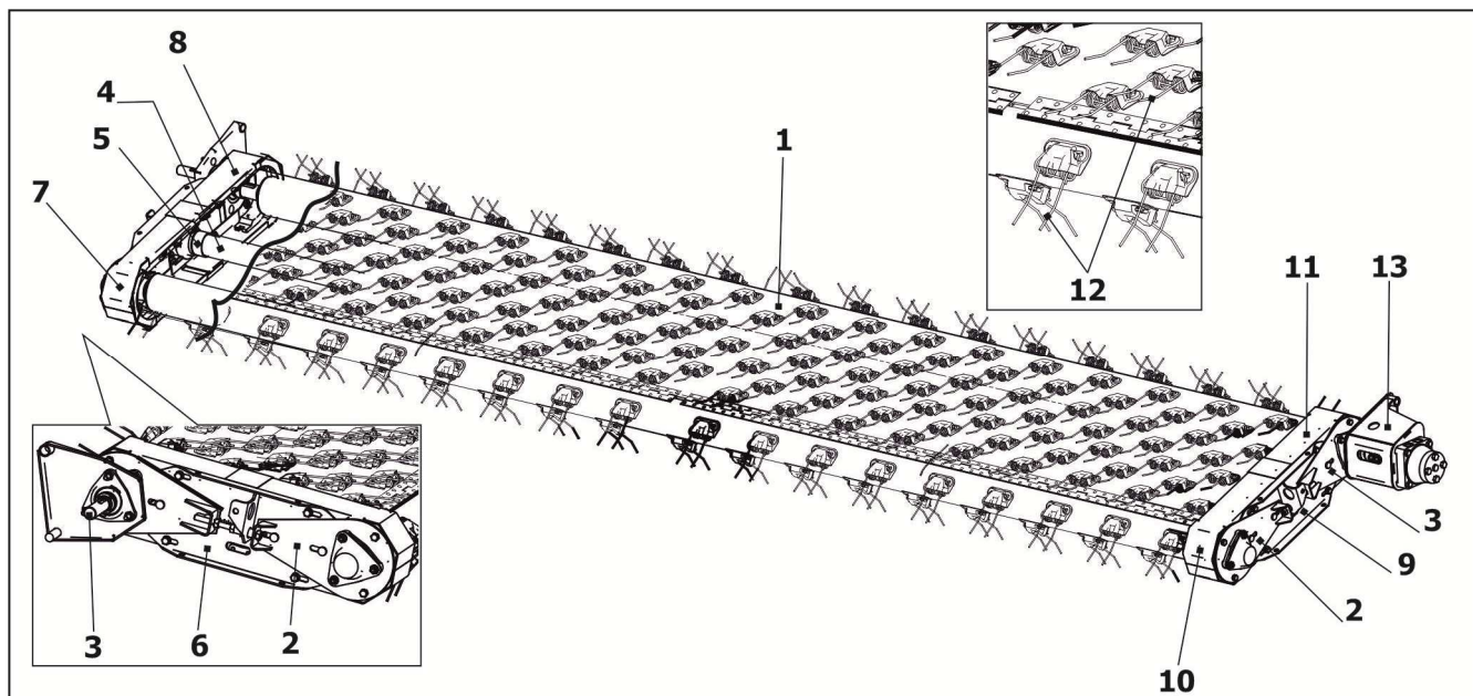
1 - полотна транспортера; 2 - вал ведомый; 3 - вал ведущий; 4 - поперечина; 5 – ролик; 6, 9 - фланец; 7, 8 – обойма; 10, 11 - обойма; 12 – палец подбирающий; 13 - гидромотор
