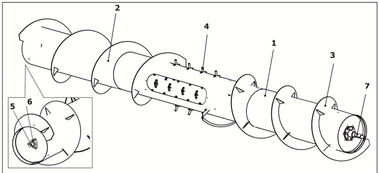
1 - труба; 2, 3 - правая и левая винтовые ленты; 4 - пальчиковый механизм; 5 - ось правая; 6 - опора; 7 - цапфа
