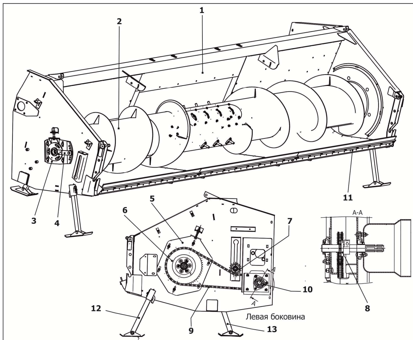
1 – каркас; 2 – шнек; 3, 5 – плита; 4 – рукоятка; 6 – муфта фрикционная предохранительная; 7 - звездочка натяжная; 8 - звездочка; 9 - цепная передача; 10 - опора; 11 - фартук стеблесьемника; 12 - передняя опора; 13 - задняя опора
