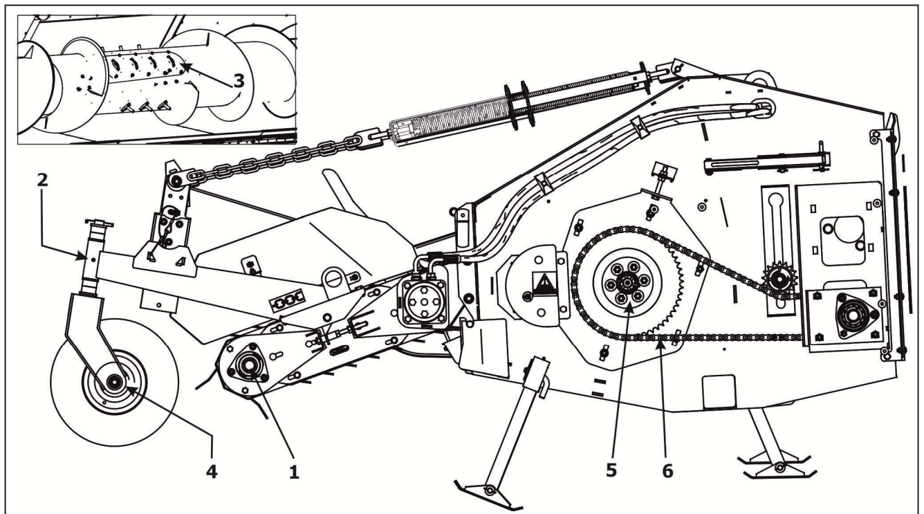
Рисунок 7.1 - Объекты смазки платформы-подборщика
