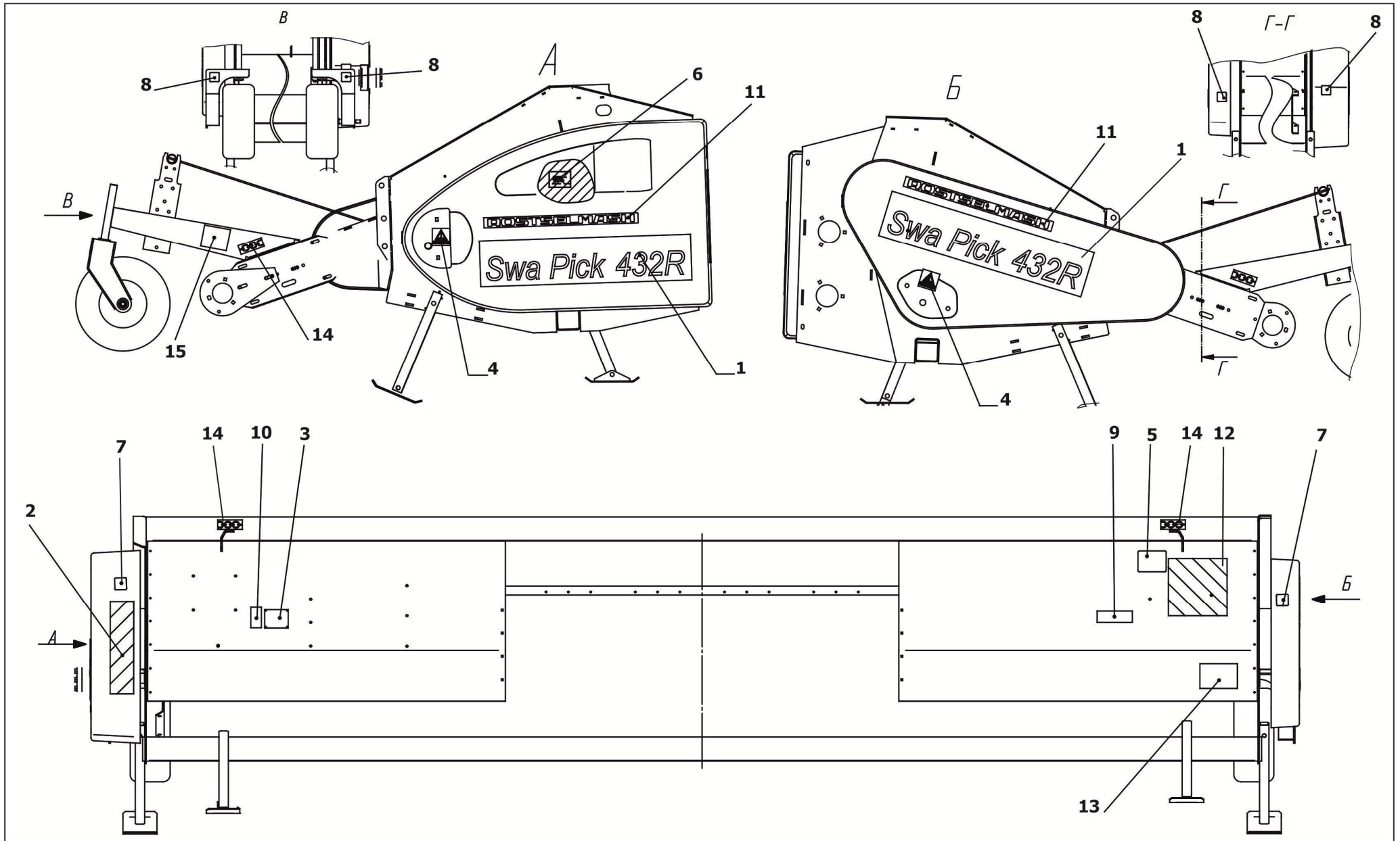
Рисунок 4.1 – Схема расположения табличек и аппликаций на платформе-подборщике
