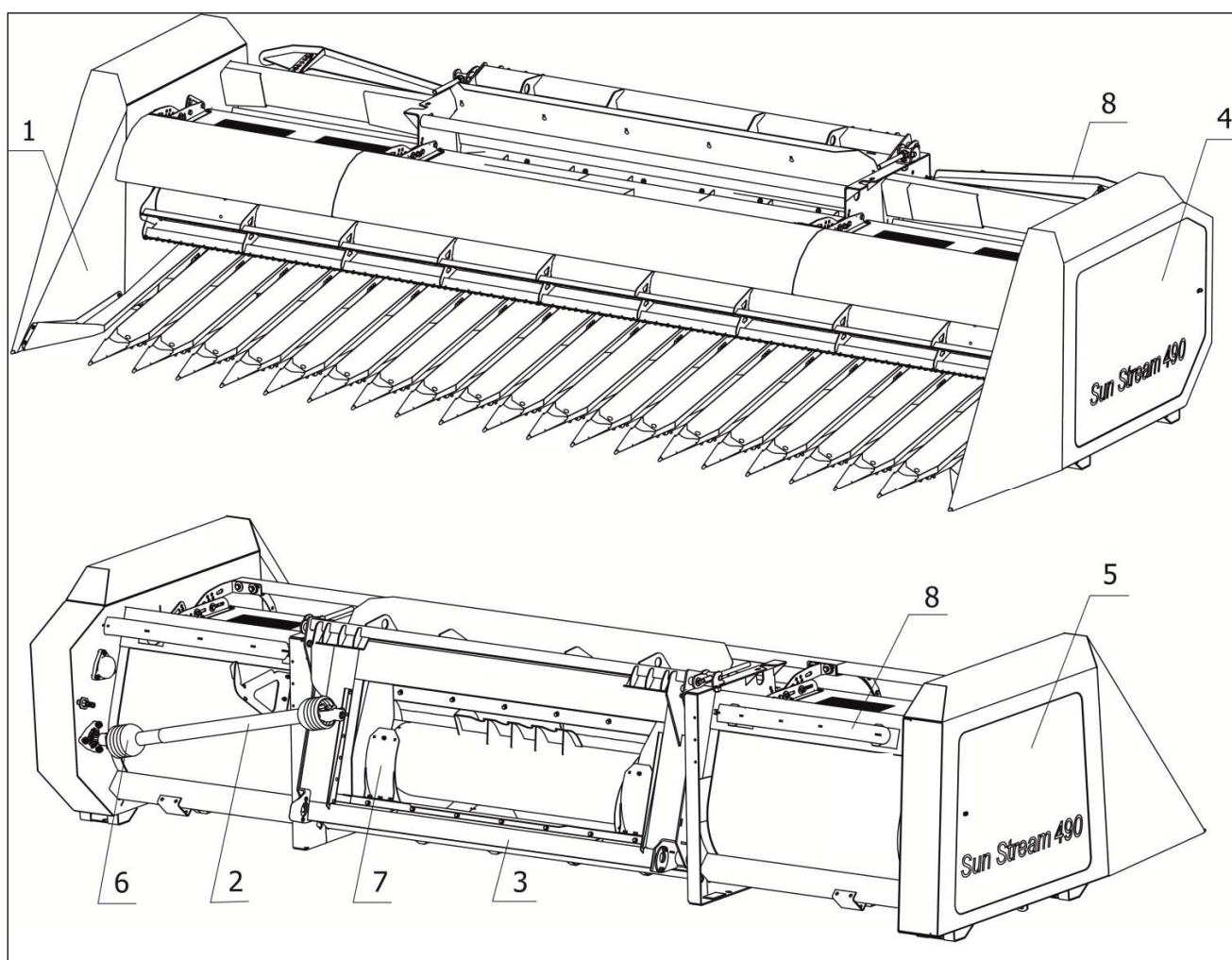
1 – Жатвенная часть; 2 – Карданная передача; 3 – Рамка переходная; 4, 5 – Защитные щитки; 6 – Кожух; 7 – Щиток; 8 – Опора
