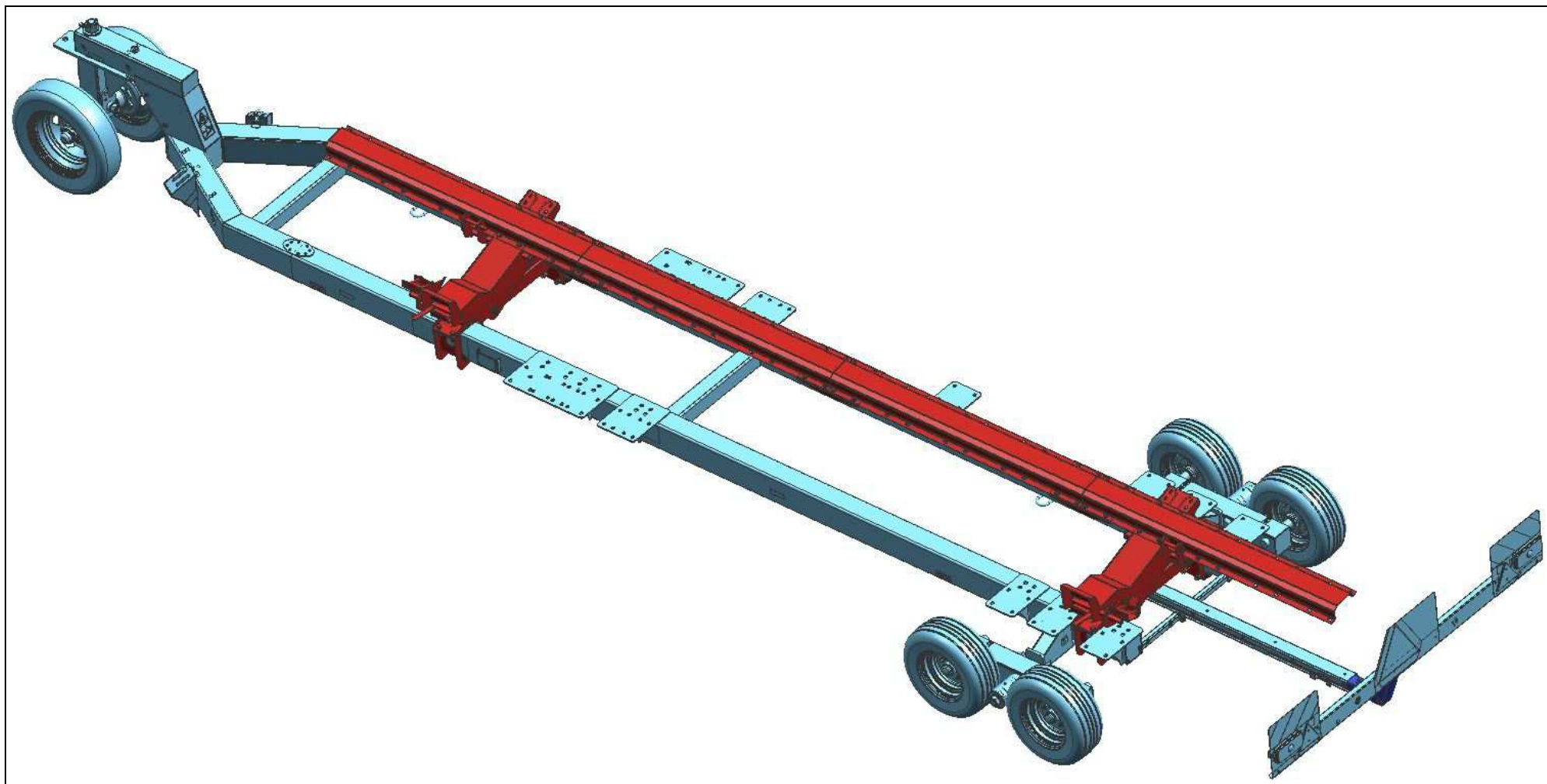
Рисунок Д.4 – Приспособление для перемещения адаптеров ППА-4000 "Uni Cart 4000" для RSM SS-560, RSM SS-650 с комплектом для транспортировки SS-780.13.00.000
