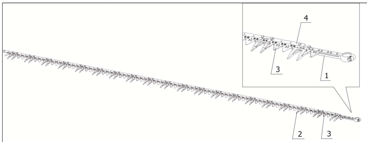
1 – Сегментно-пальцевый брус; 2 – Двойной палец; 3 – Нож; 4 – Пластина трения
