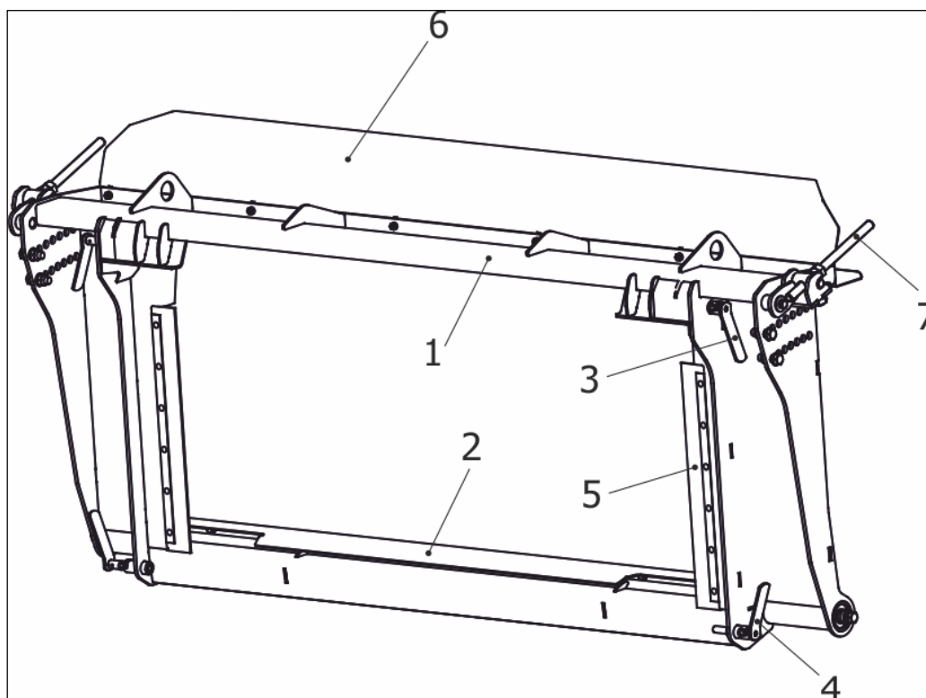
1 – Рамка переходная; 2 – Уголок; 3, 4 – Шкворень; 5 – Уплотнитель; 6 – Козырек; 7 - Тяга
