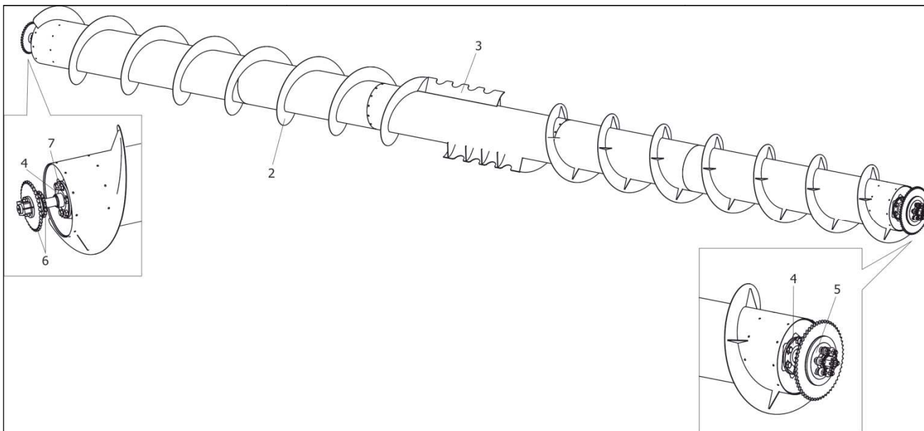
1 – Корпус; 2 – Спираль; 3 – Лопатка; 4 – Цапфа; 5 – Предохранительная муфта; 6 – Блок-звёздочка; 7 – Прокладка регулировочная Рисунок 2.9 - Шнек
