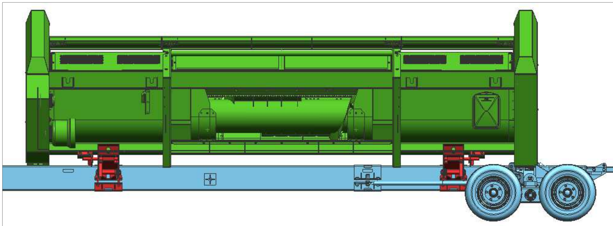
Рисунок Д.5 - Приспособление модульное для перемещения адаптеров ПМА-4000 «Pro Cart 4000» с установленной жаткой RSM SS-490 (SS-560) и комплектом для транспортировки SS-490.23.00.000 (SS-490.23.00.000-01)
