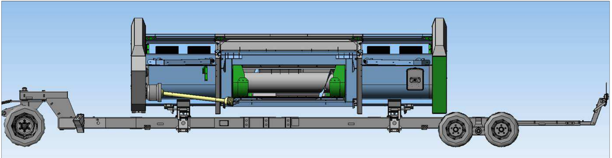
Рисунок Д.1 – Приспособление для перемещения адаптеров ППА-4000 "Uni Cart 4000" с установленной жаткой RSM SS-490 с комплектом для транспортировки SS-490.13.00.000А Вид сбоку
