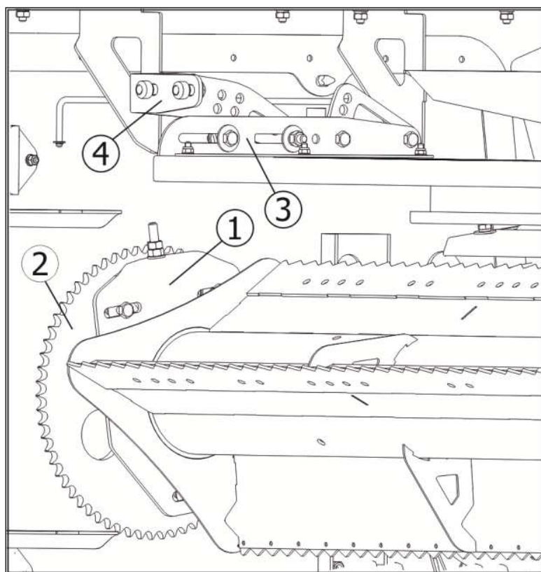
1 - Опора; 2 – Звездочка; 3, 4 – Рычаг
