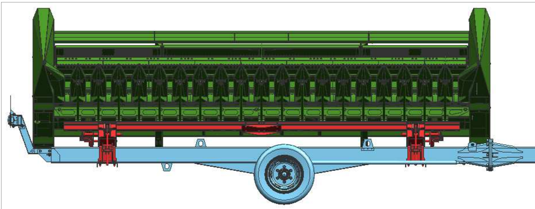
Рисунок Д.7 - Приспособление для перемещения адаптеров ППА-700 «Uni Cart 3000» с установленной жаткой RSM SS-490 (SS-560) и комплектом для транспортировки SS-490.23.00.000-02 (SS-490.23.00.000-03)
