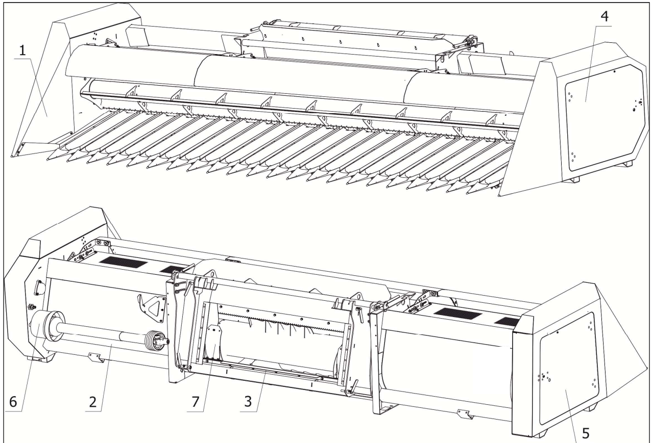
1 – Жатвенная часть; 2 – Карданная передача; 3 – Рамка переходная; 4, 5 – Защитные щитки; 6 – Кожух; 7 – Щиток
