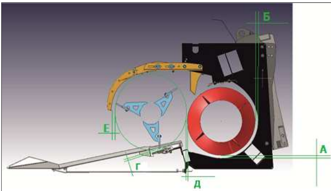
Рисунок 5.1- Регулировка жатки
