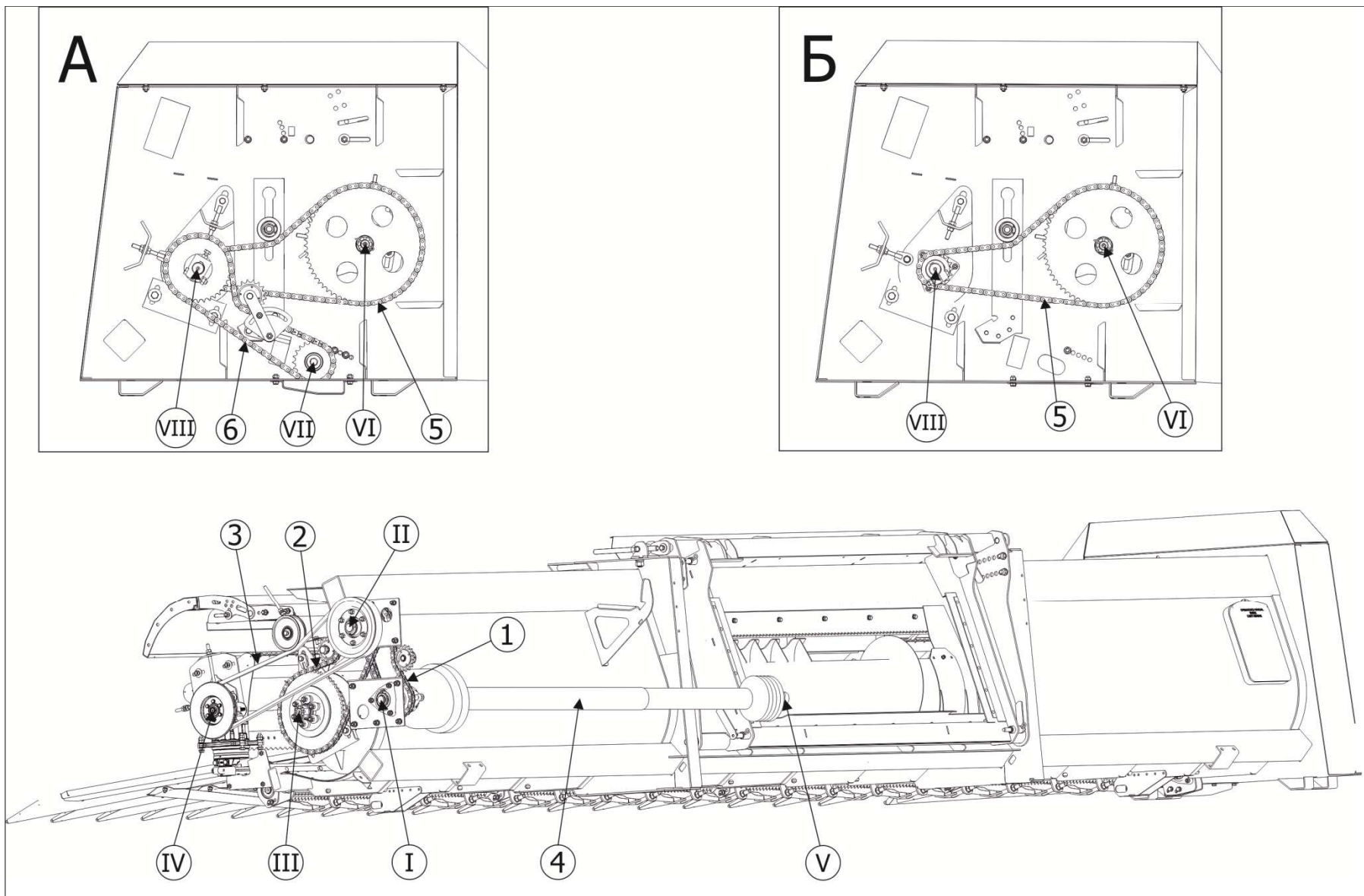
- Схема передач жатки
