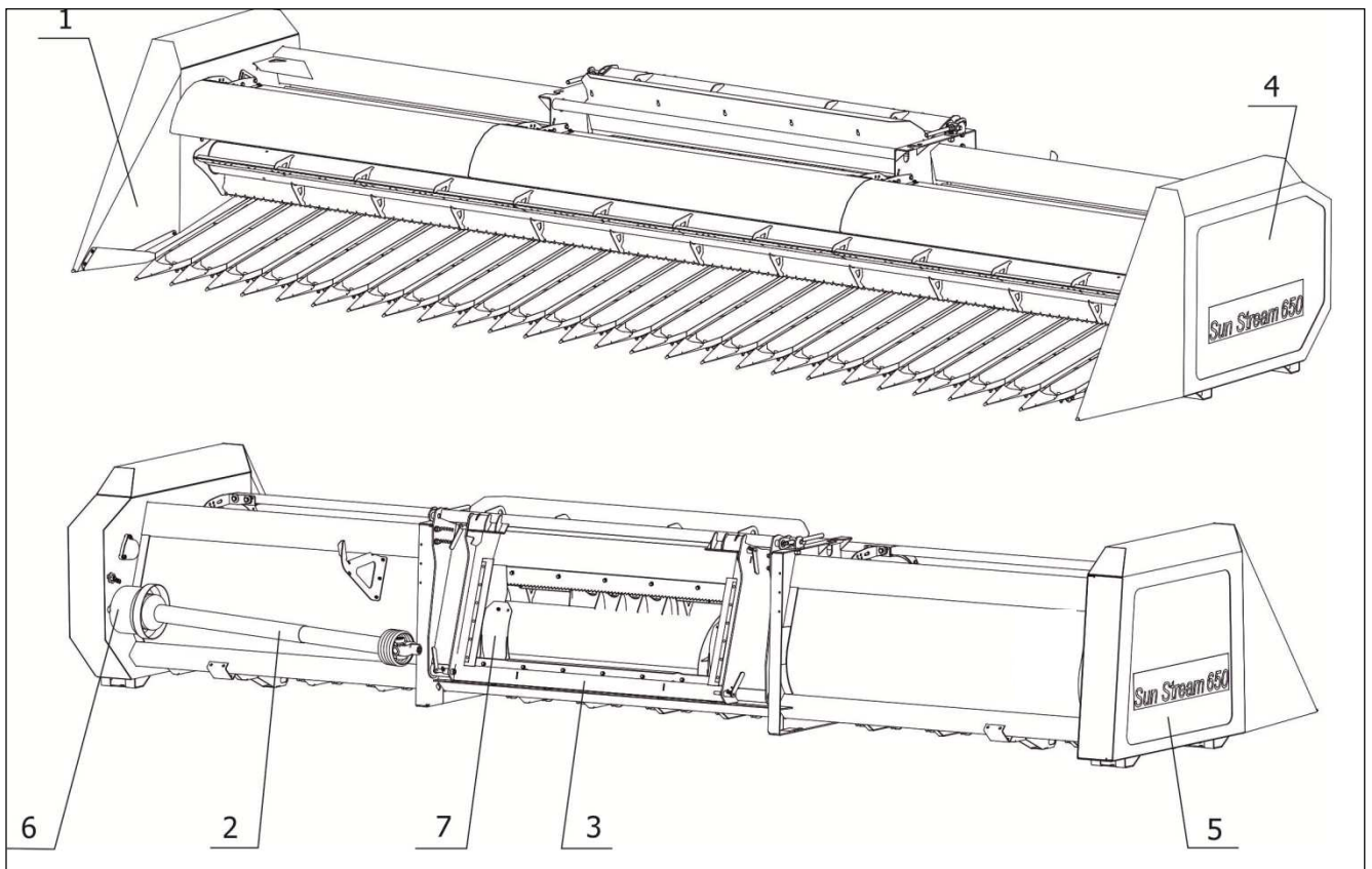
1 – Жатвенная часть; 2 – Карданная передача; 3 – Рамка переходная; 4, 5 – Защитные щитки; 6 – Кожух; 7 – Щиток
