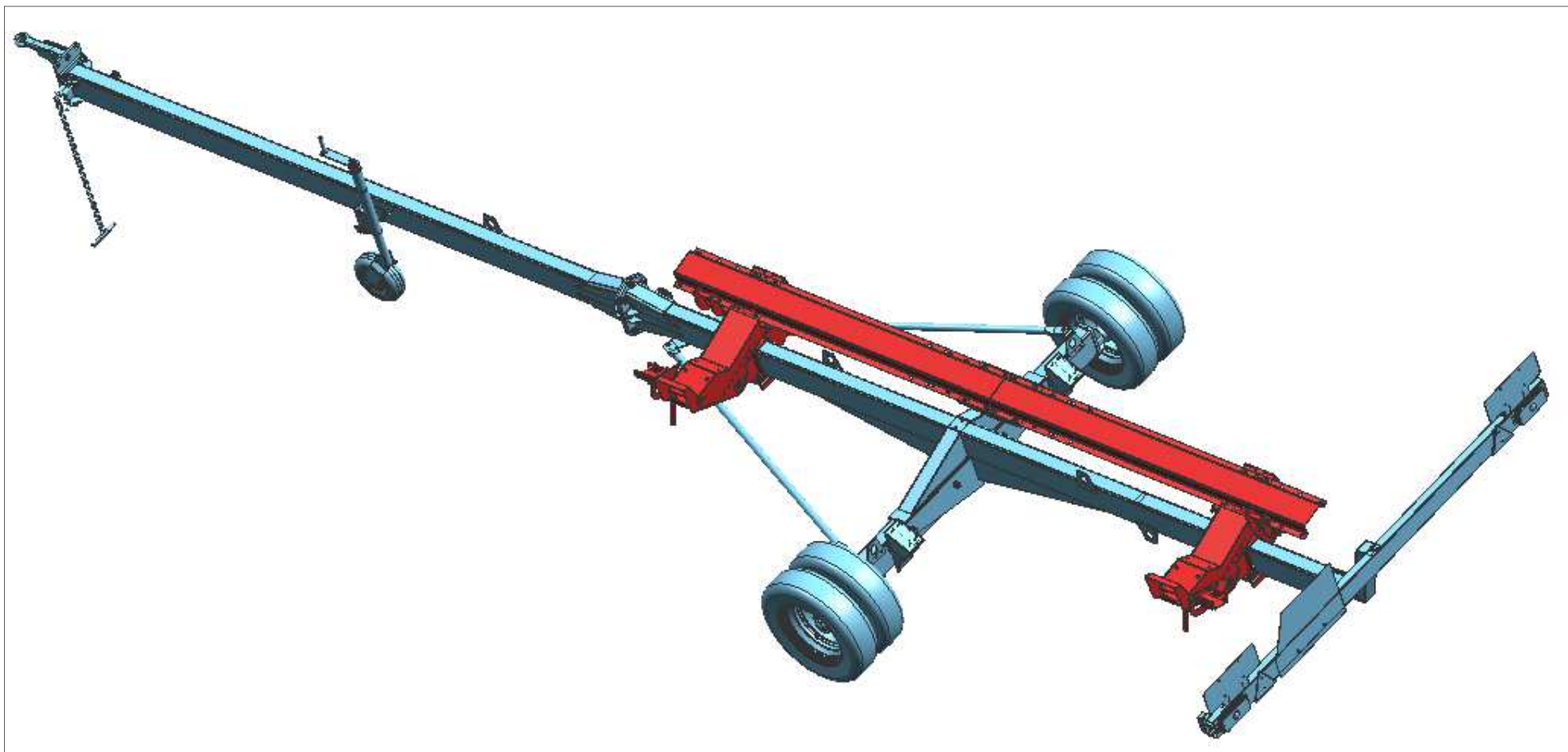
Рисунок Д.8 - Приспособление для перемещения адаптеров ППА-700 «Uni Cart 3000» для жатки RSM SS-490 (SS-560) с комплектом для транспортировки SS-490.23.00.000-02 (SS-490.23.00.000-03)
