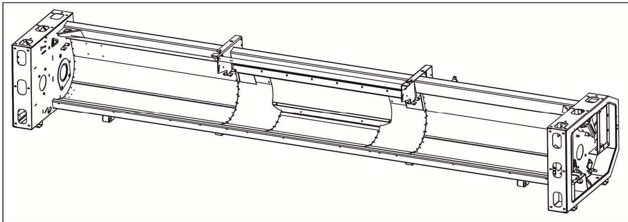
Рисунок 2.5 - Рама
