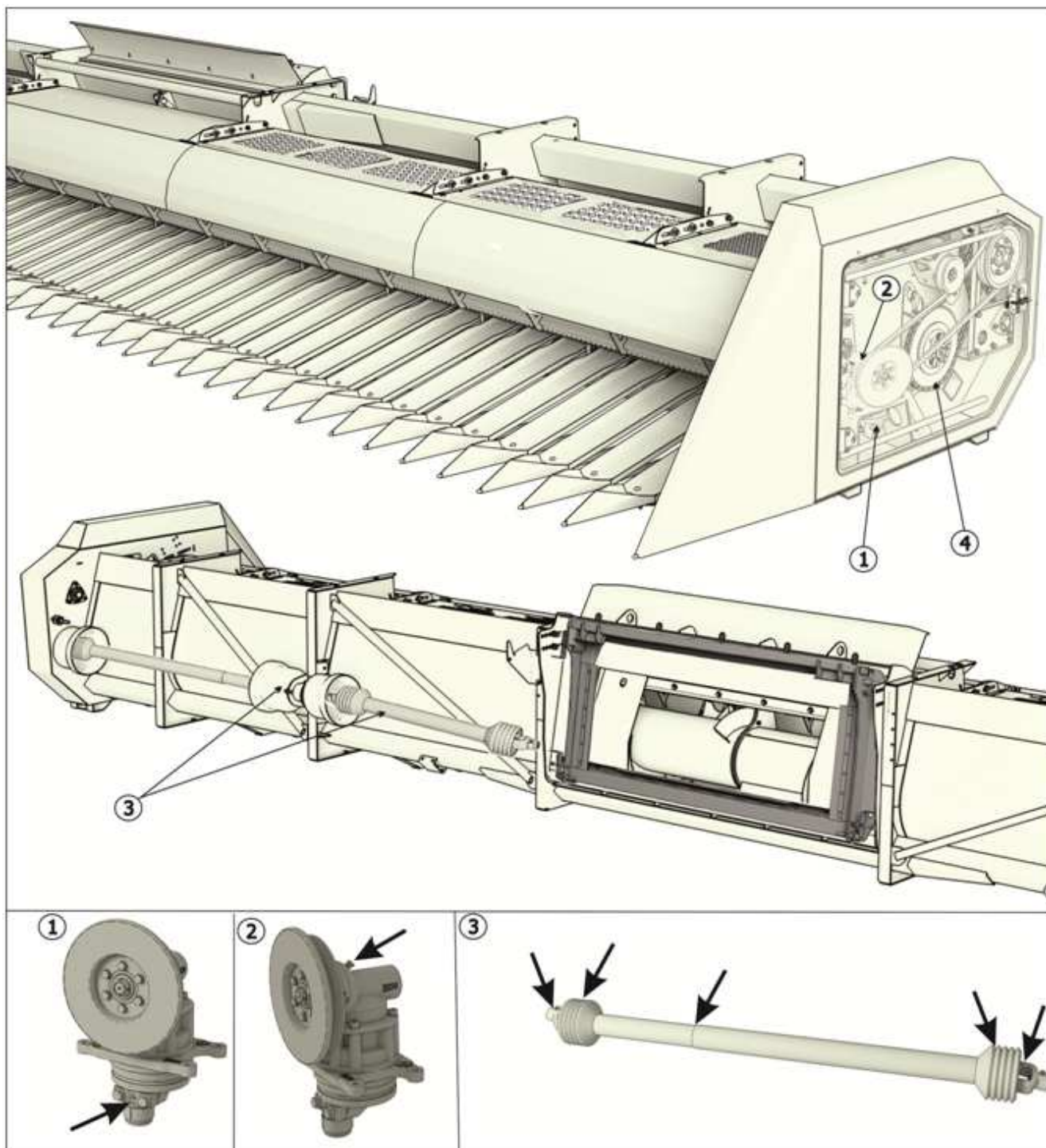
Рисунок 6.1 – Смазка жатки
