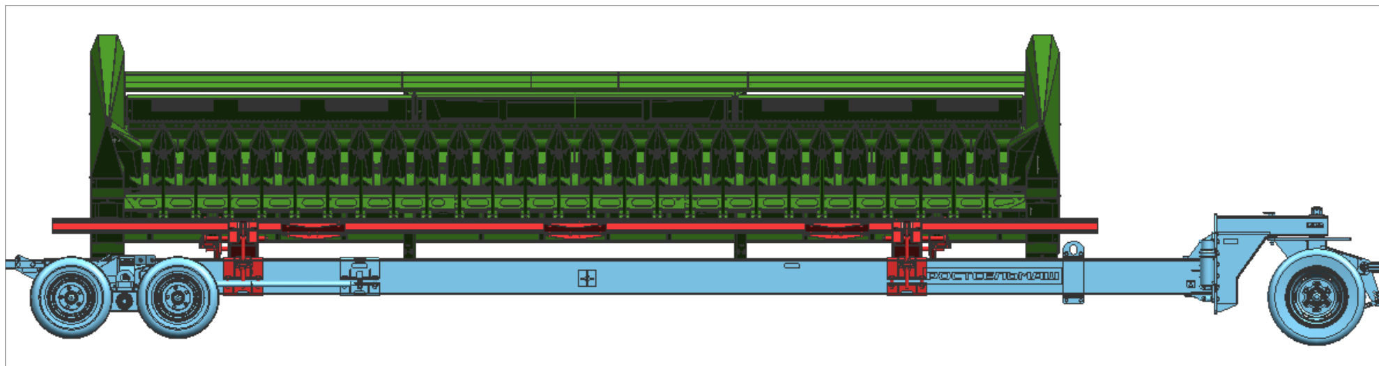
Рисунок Д.9 - Приспособление модульное для перемещения адаптеров ПМА-4000 «Pro Cart 4000» с установленной жаткой RSM SS-650 и комплектом для транспортировки SS-780.23.00.000
