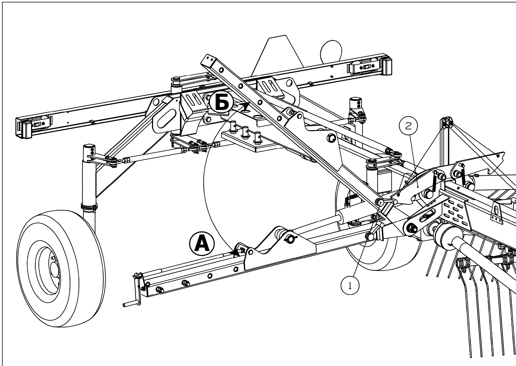
А, Б – Положение грабли 1 - Упор балки; 2 - Зацеп Рисунок 5.2
