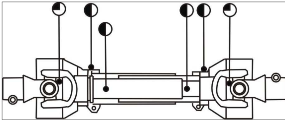
Рисунок 8.2 - Места смазки карданного вала
