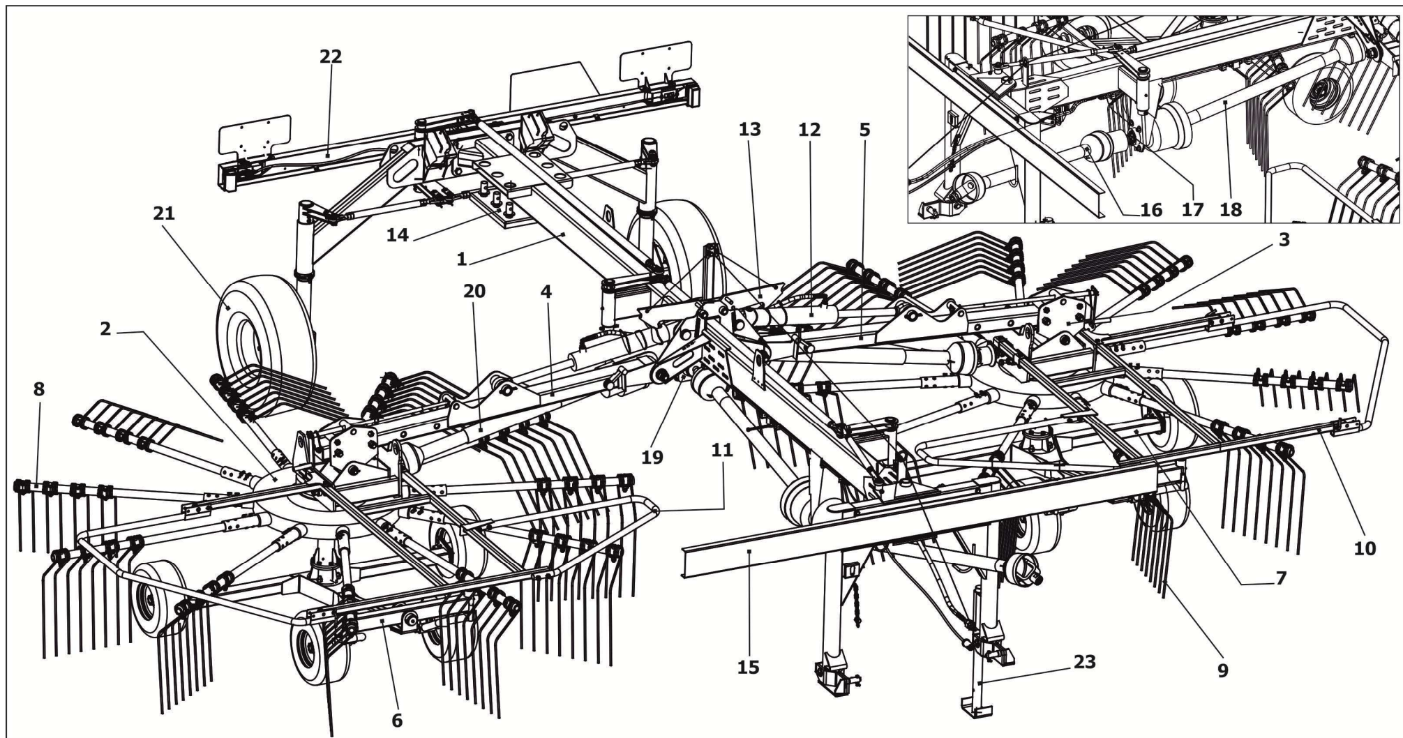
1 - Балка средняя; 2, 3 - Ротор; 4, 5 - Балка ротора; 6, 7 - Шасси тележки; 8, 9 - Граблина; 10, 11 - Ограждение; 12 - Гидроцилиндр; 13 - Зацеп; 14 - Кронштейн; 15 - Навеска; 16, 18, 20 - Вал карданный; 17 - Привод; 19 - Редуктор конический; 21 - Колесо; 22 - Балка задняя; 23 - Опора
