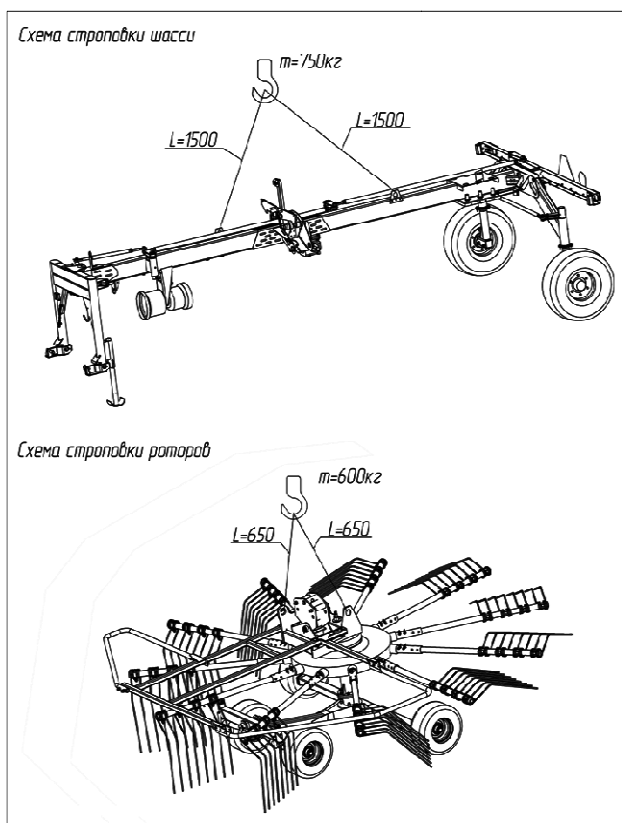
Рисунок 9.1 – Аппликация «Схема строповки»
