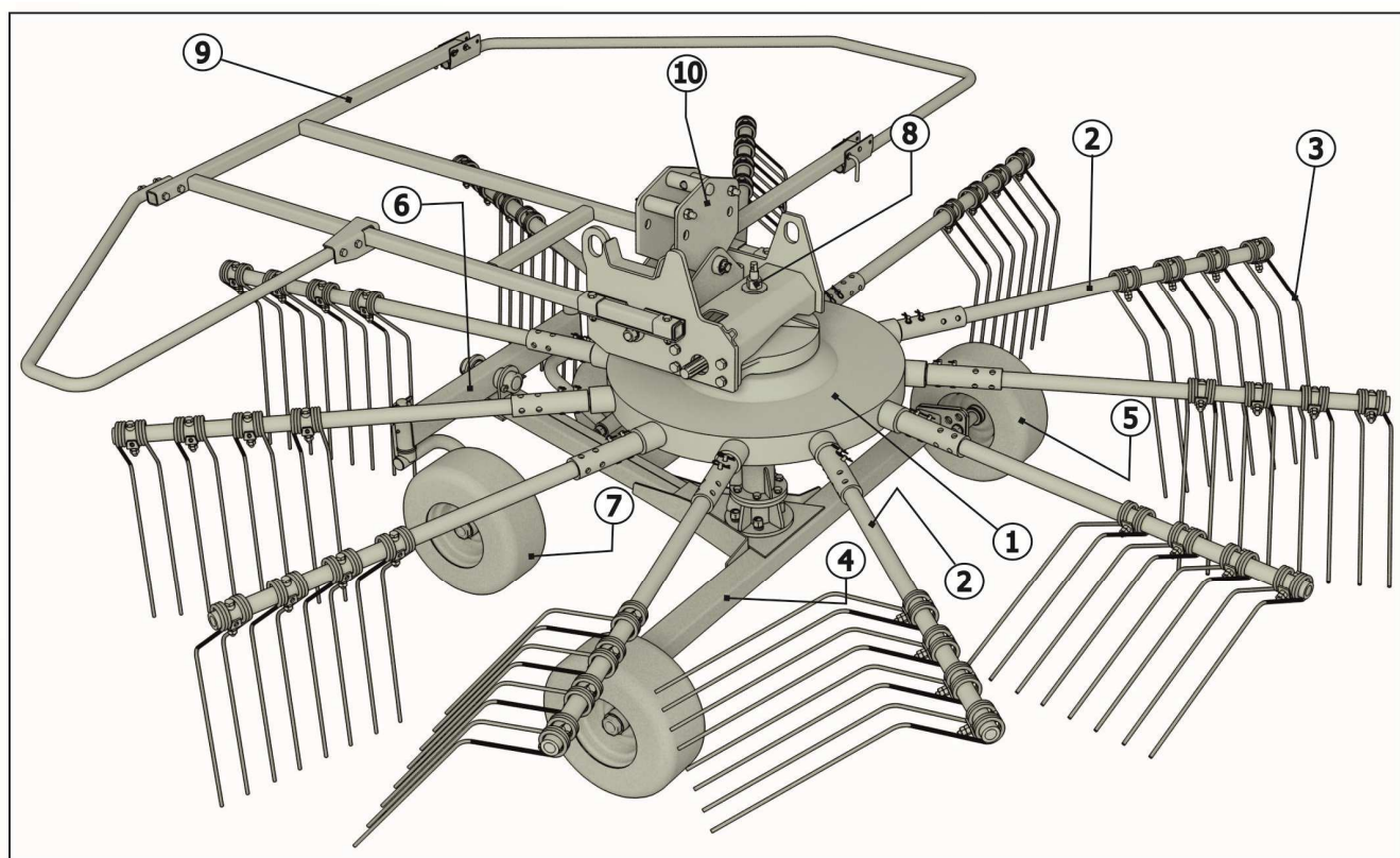
1 - Редуктор; 2 - Штанга; 3 - Граблина; 4 - Сница; 5 - Колесо заднее; 6 - Балка передняя; 7 - Колесо переднее (флюгерное); 8 - Винт регулировочный; 9 - Ограждение; 10 - Подвеска;
