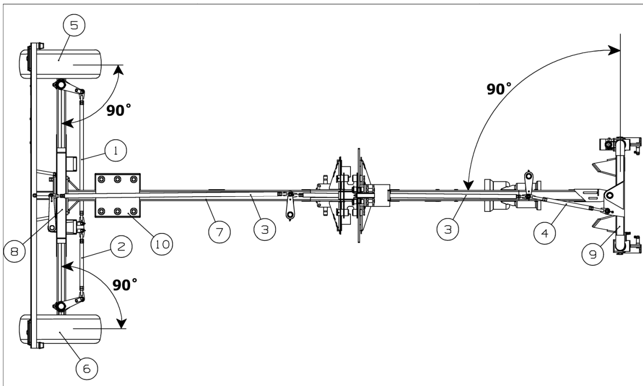
1, 2, 3, 4 - Тяга; 5,6- Колесо ходовое; 7 - Балка средняя; 8 - Балка задняя; 9 – Навеска; 10 - Кассетница Рисунок 6.2 - Регулировка прямолинейности хода граблей
