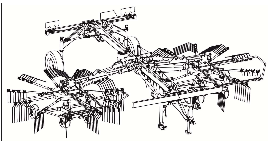
Рисунок 1.1 – Грабли роторные прицепные ГРП-810 «Kolibri Duo»
