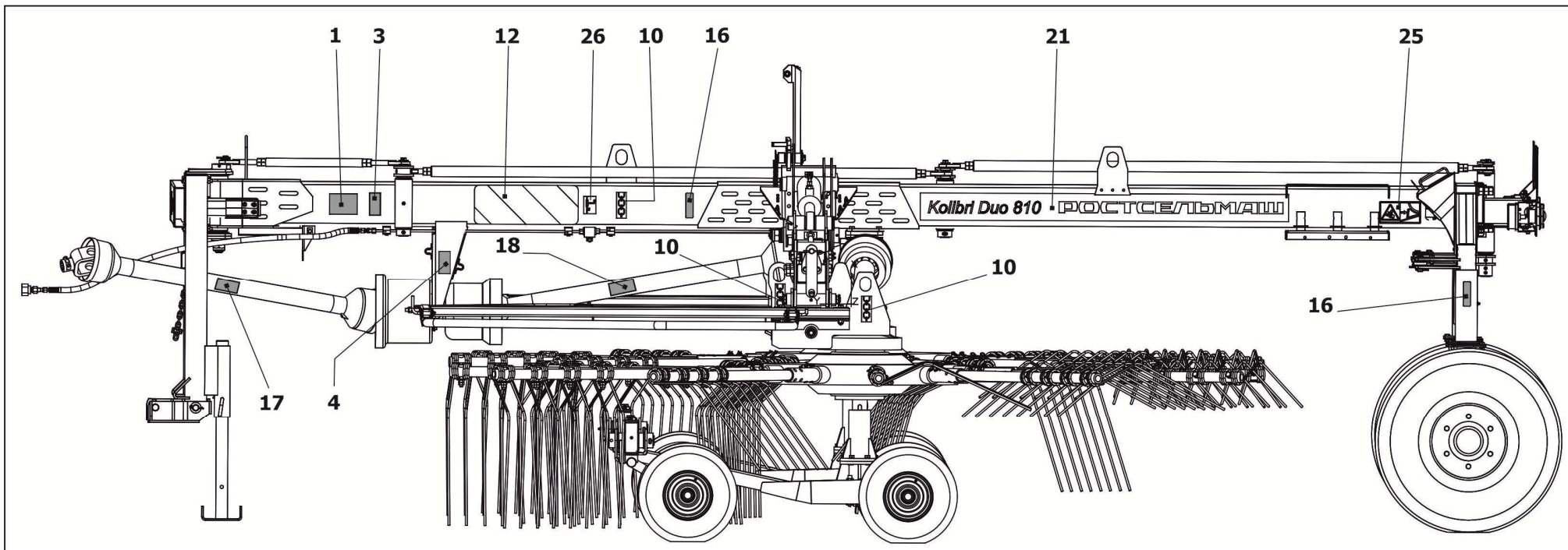
Рисунок 4.2 – Месторасположение табличек и аппликаций на граблях
