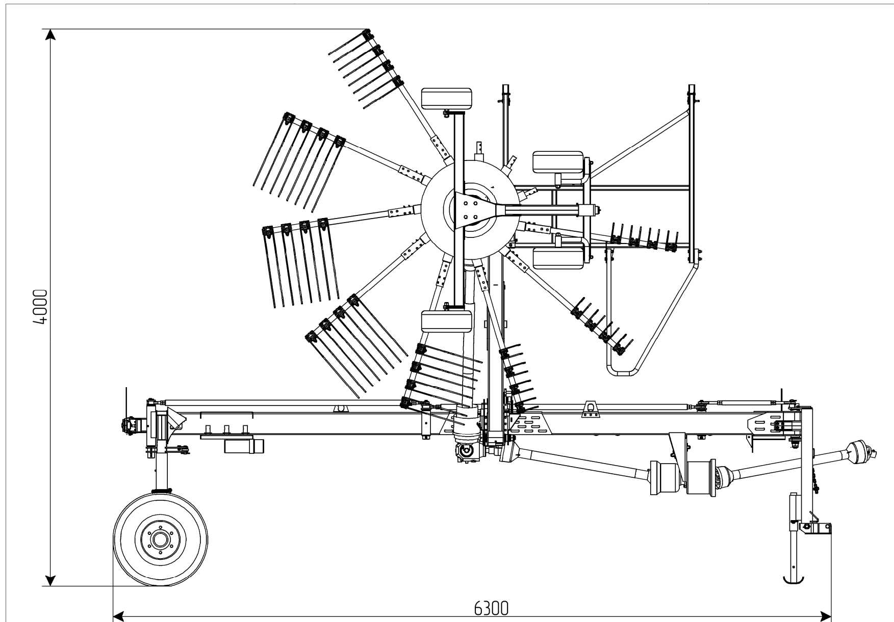
Рисунок 2.1 - Габаритные размеры граблей в транспортном положении
