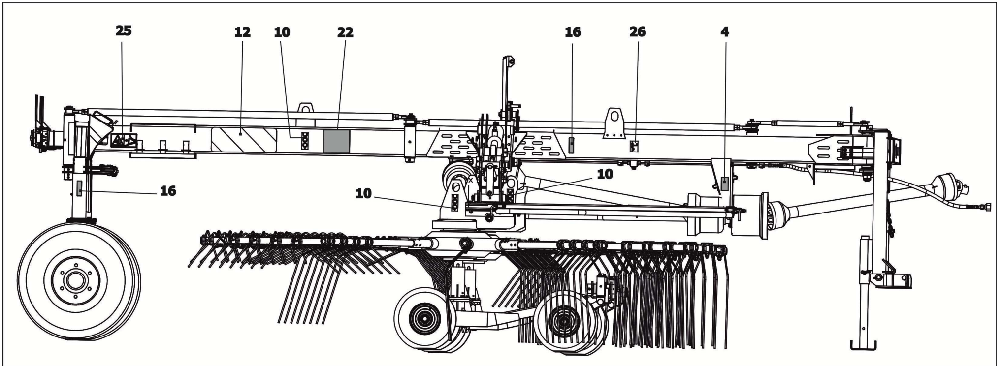
Рисунок 4.1 – Месторасположение табличек и аппликаций на граблях
