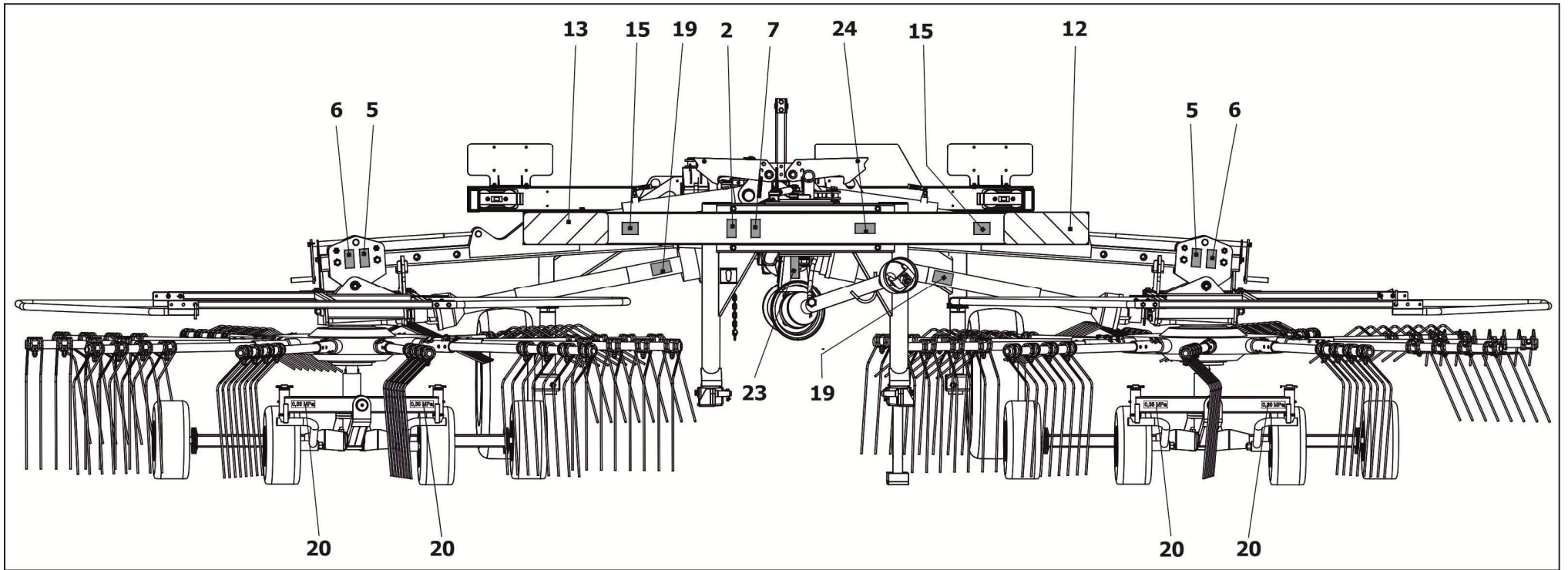
Рисунок 4.4 – Месторасположение табличек и аппликаций на граблях
